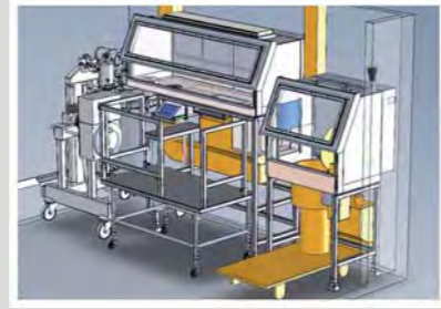
Befüllen Konustrockner
